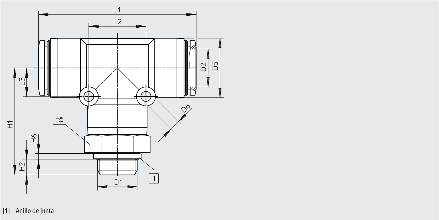
Dimensiones – Racor rápido en T QST-...-16, rosca G con anillo de junta
