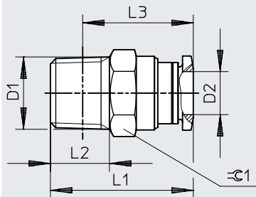
Dimensiones – Racor rápido roscado QS-...-I, rosca R
